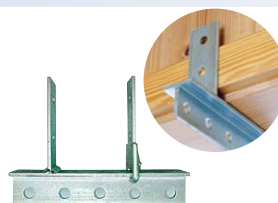
PROMO Bovenbevestiger verstelbaar, voor hangnylons en ketting / Regelbaar voor verschillende breedte van de balk zolang de voorraad strekt Art. Nr. 02 286-1 € 9,50
